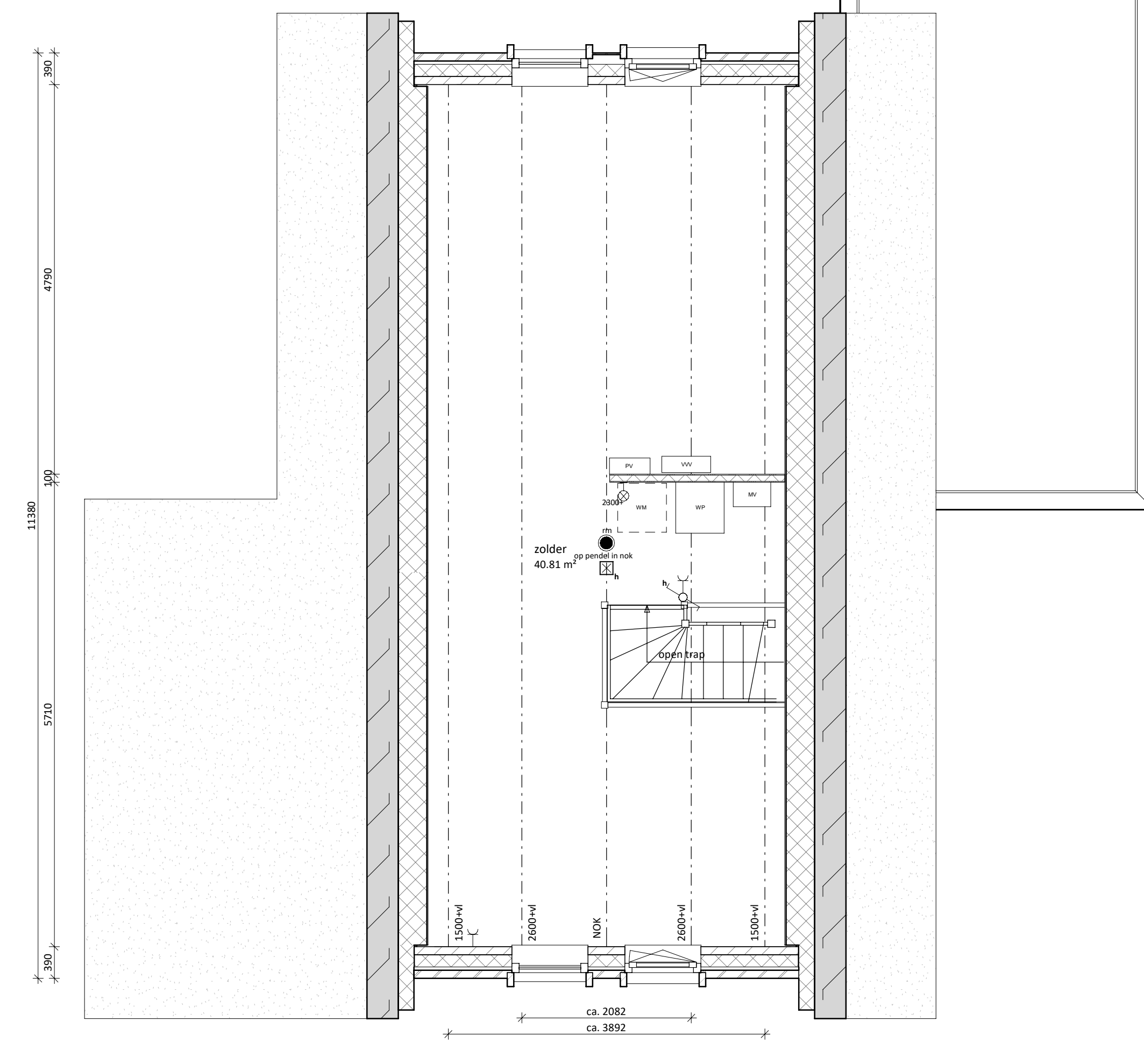
tweede verdieping 1:50
