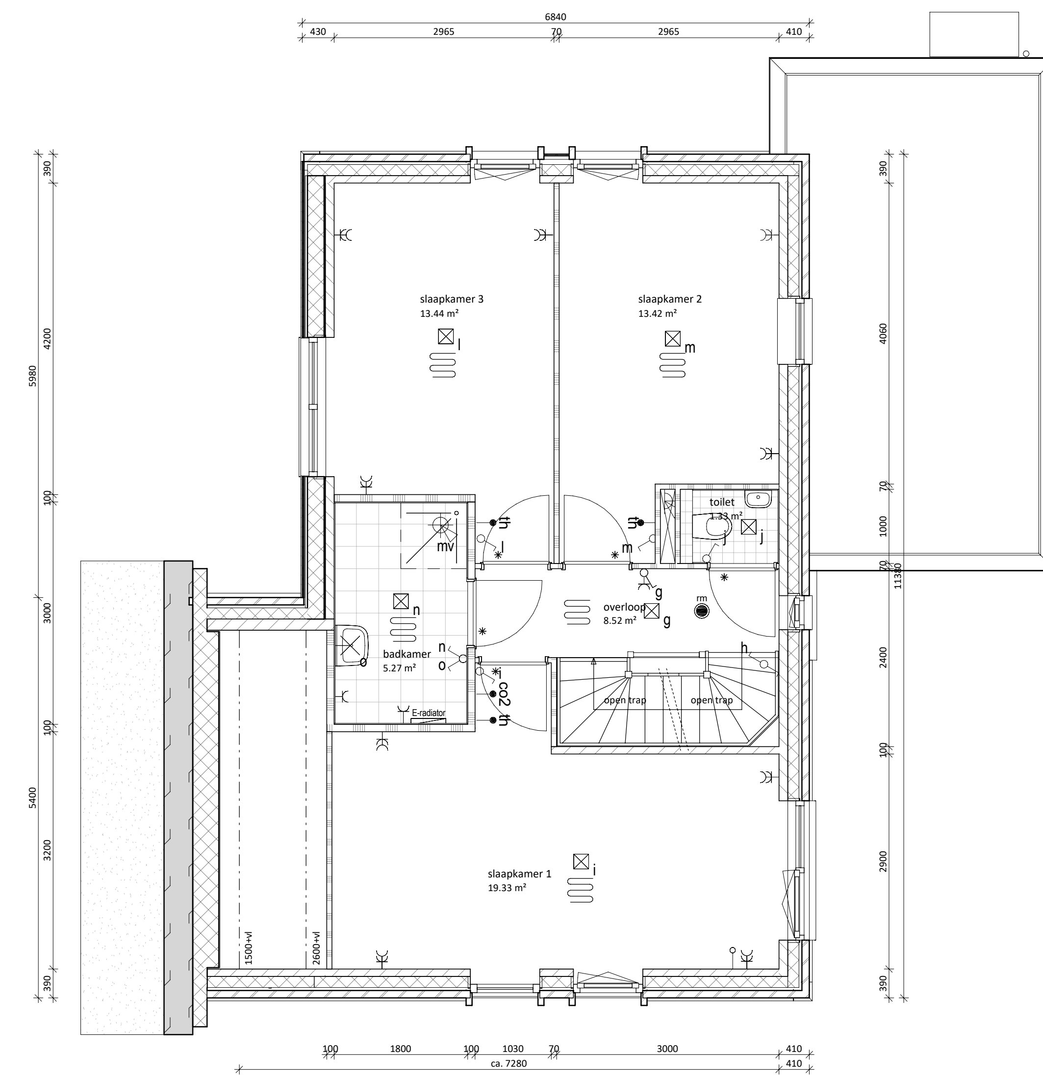
eerste verdieping 1:50
