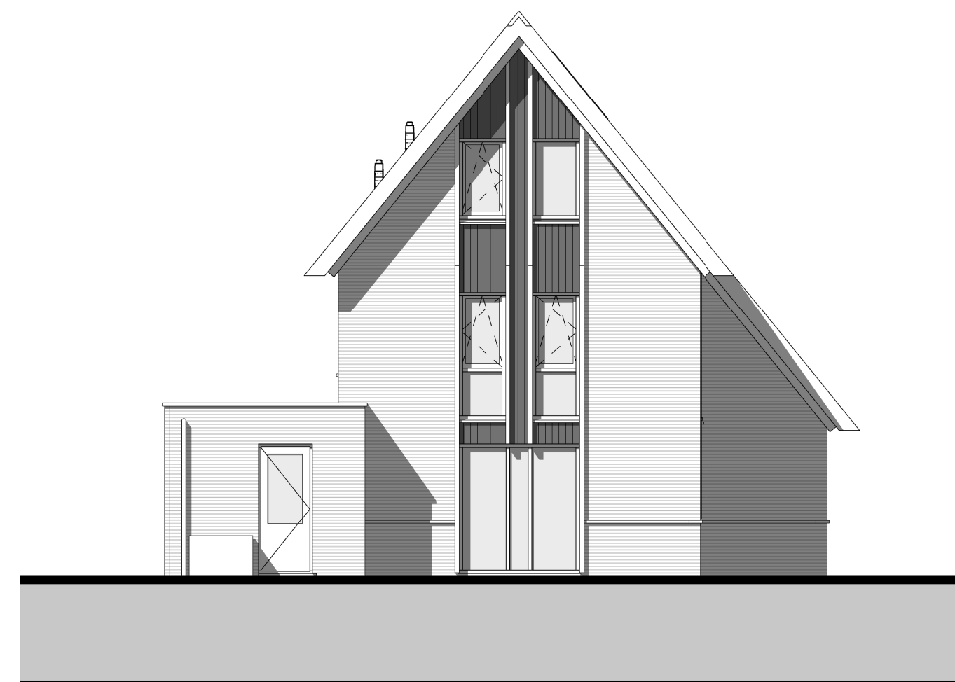
achtergevel 1:100
