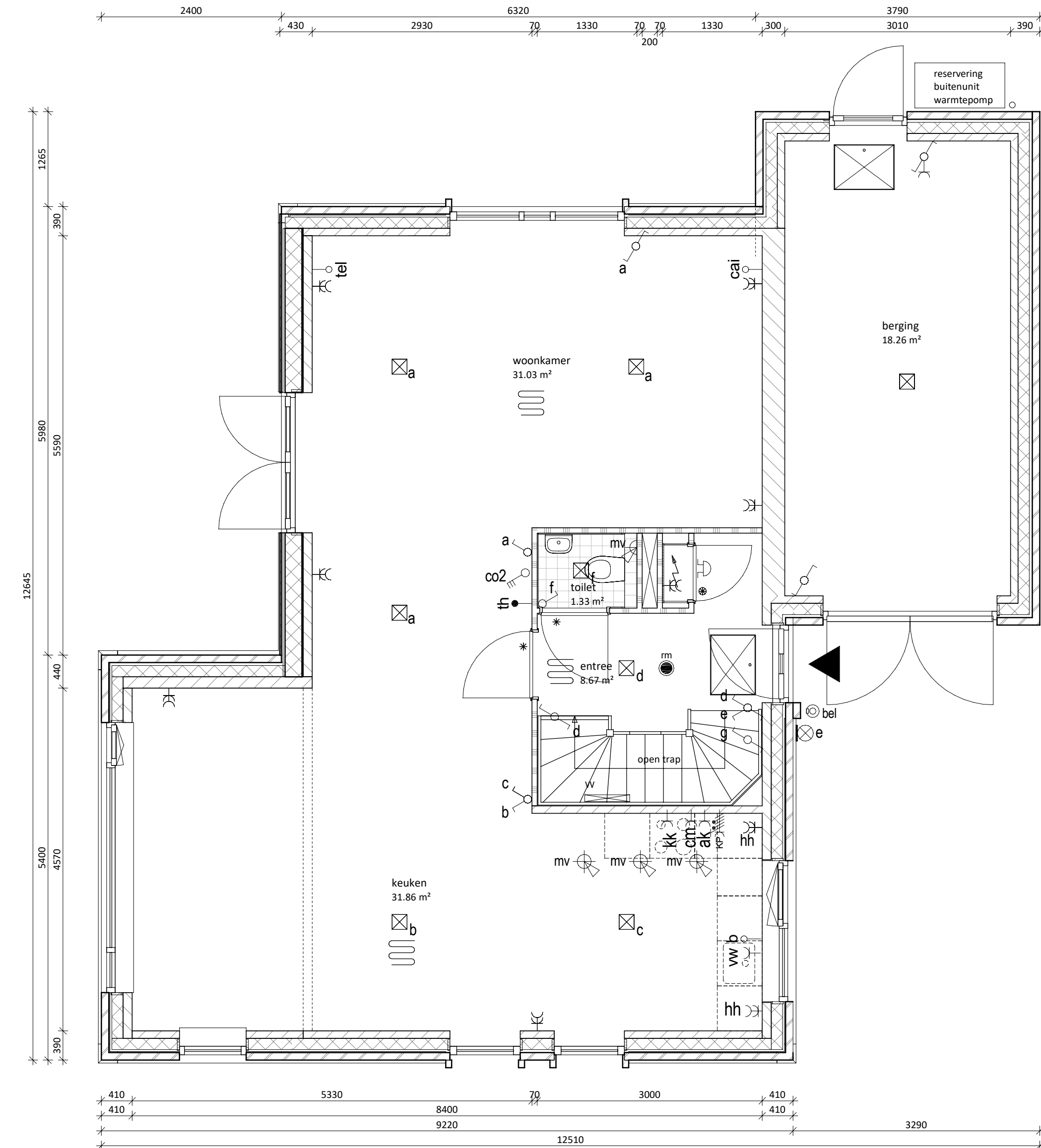
begane grond 1:50
