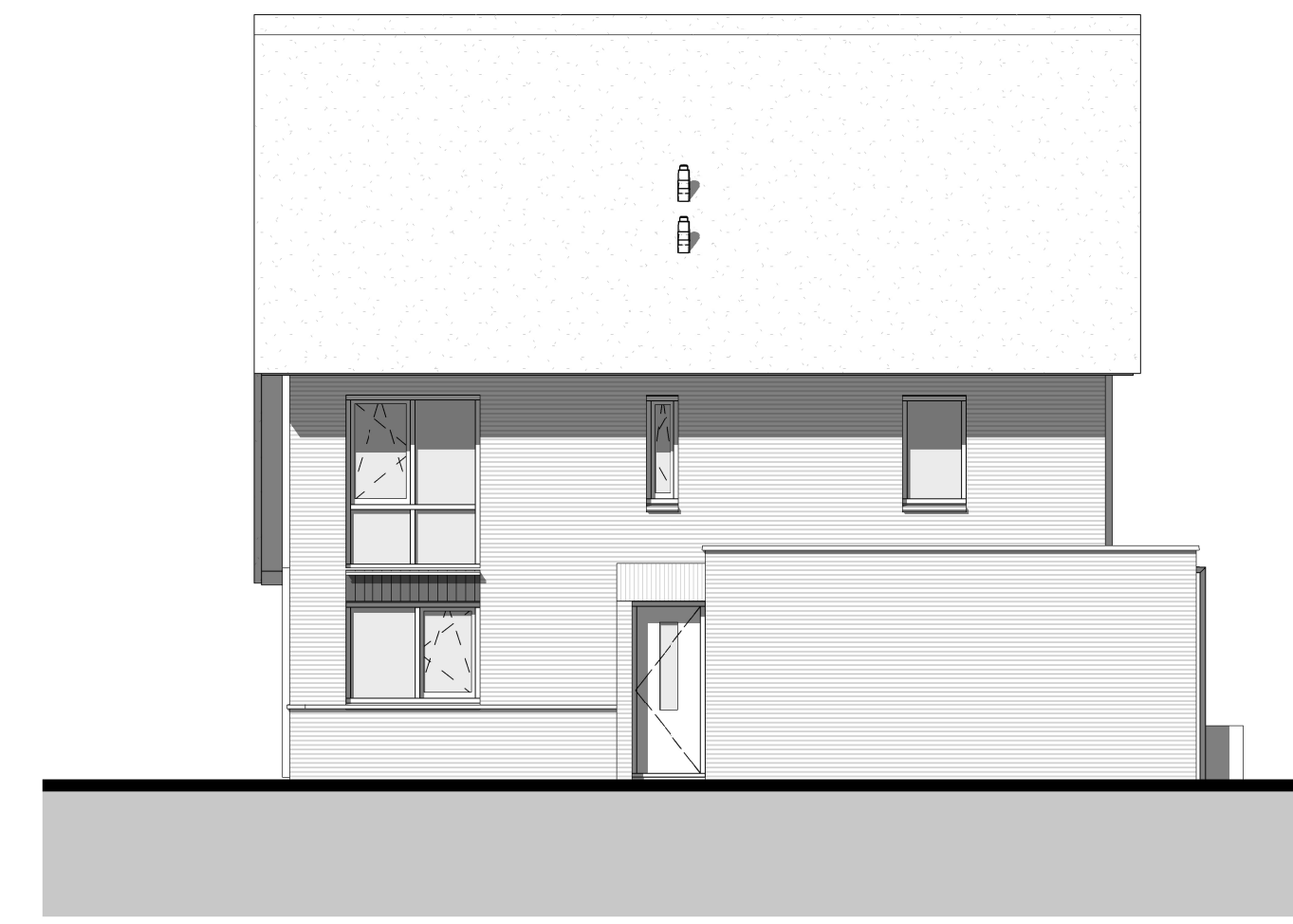
rechterzijgevel 1:100
