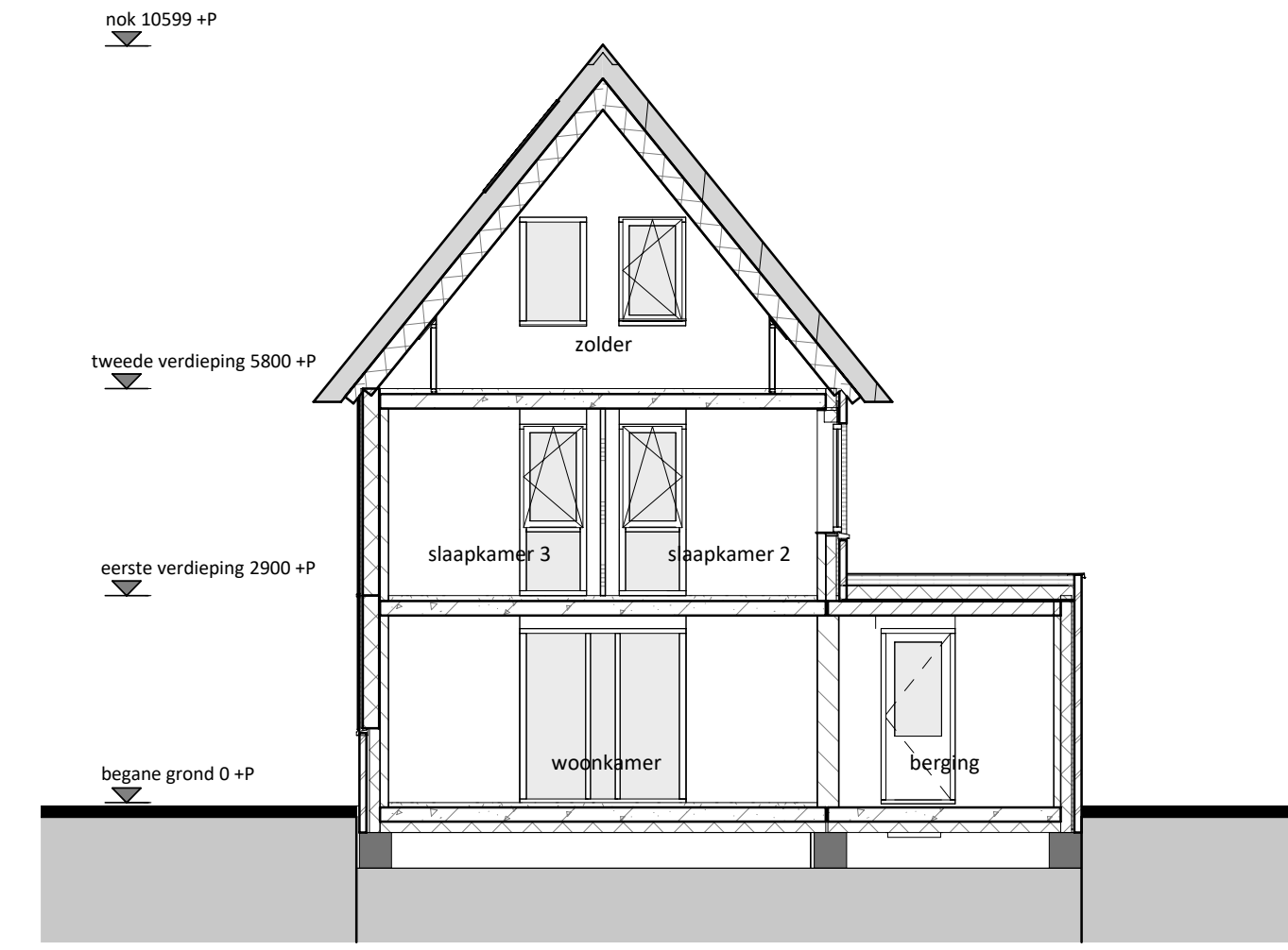
doorsnede 1:100
