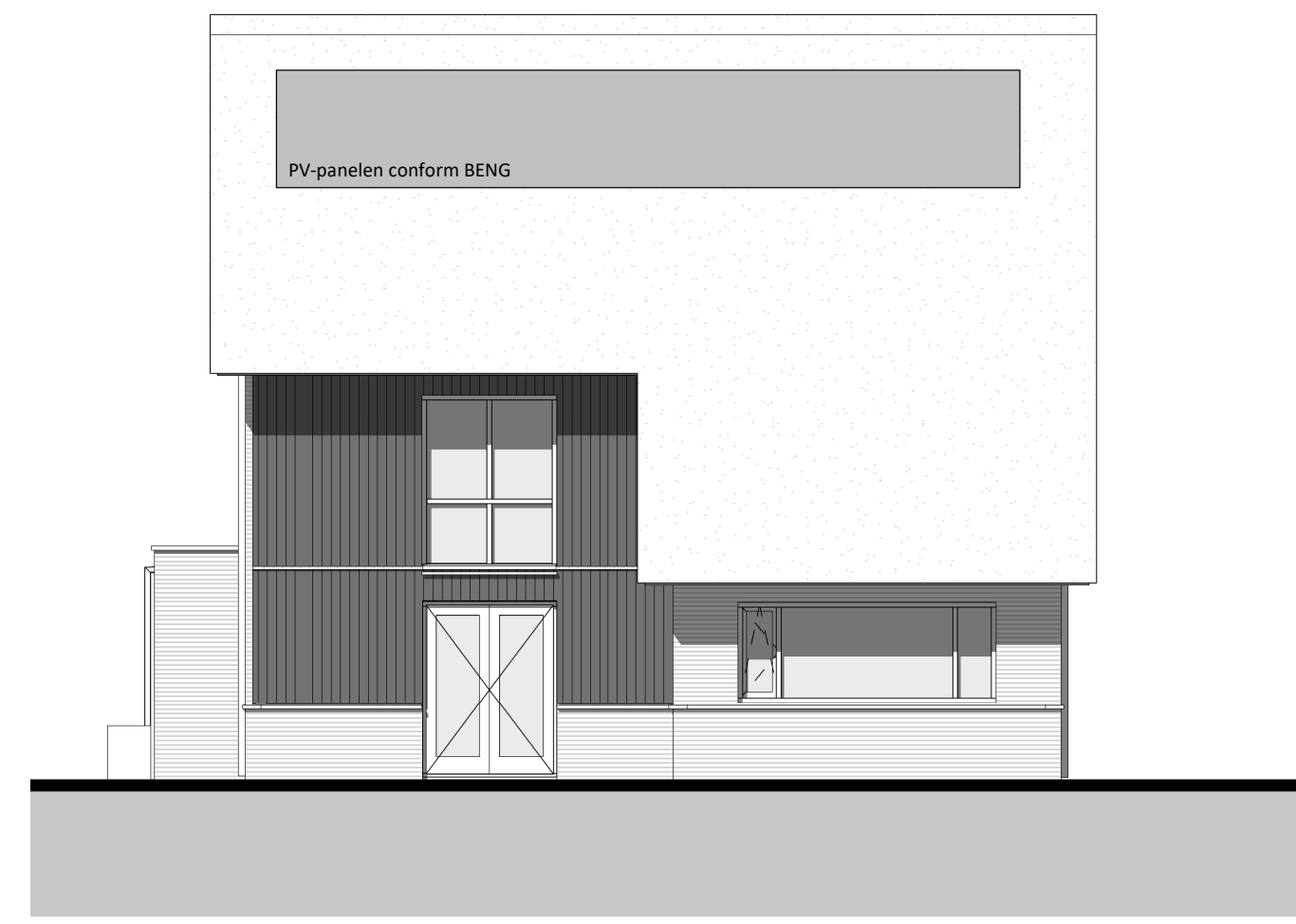
linkerzijgevel 1:100
