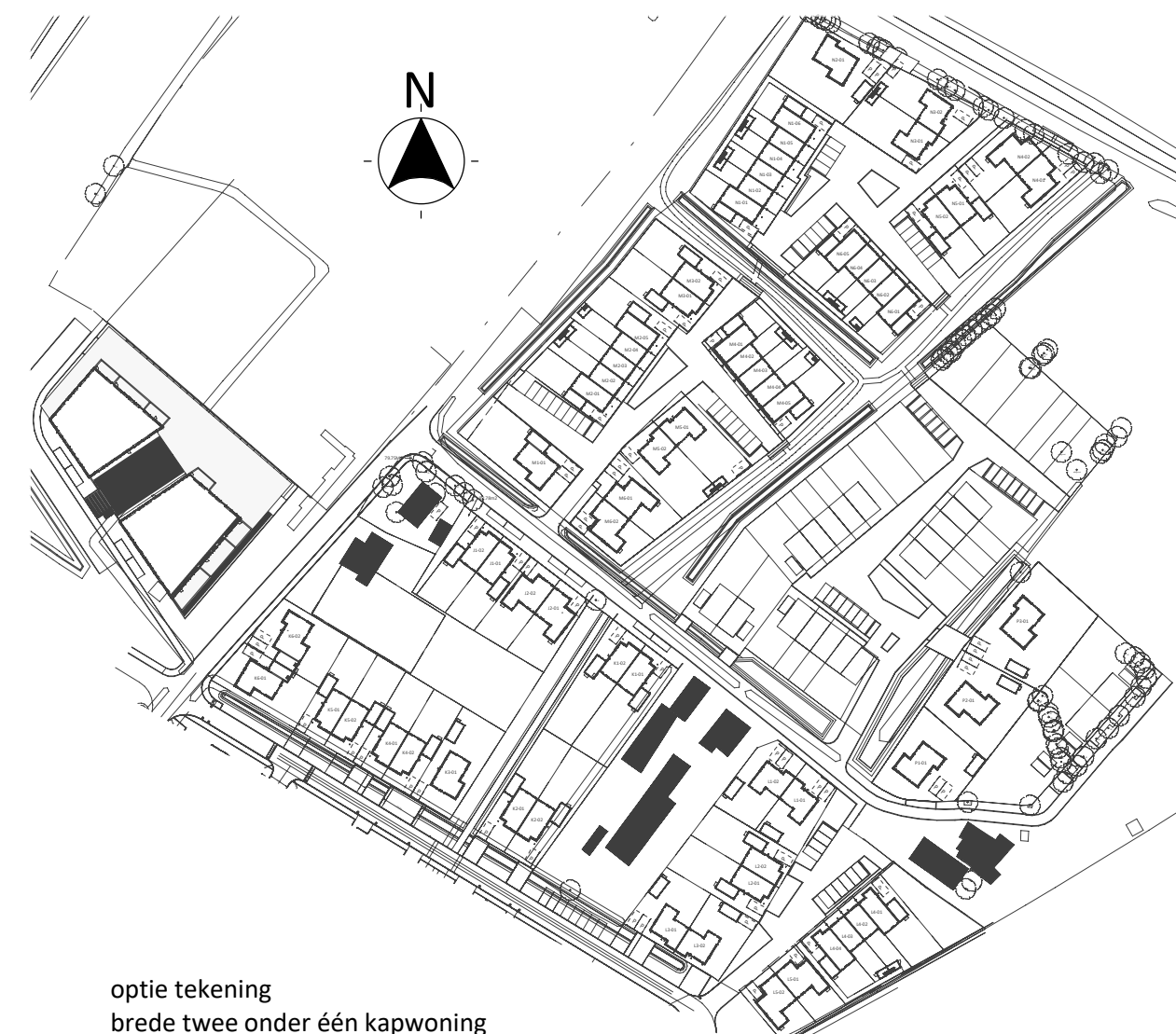
optie tekening brede twee onder één kapwoning type M5, N3
