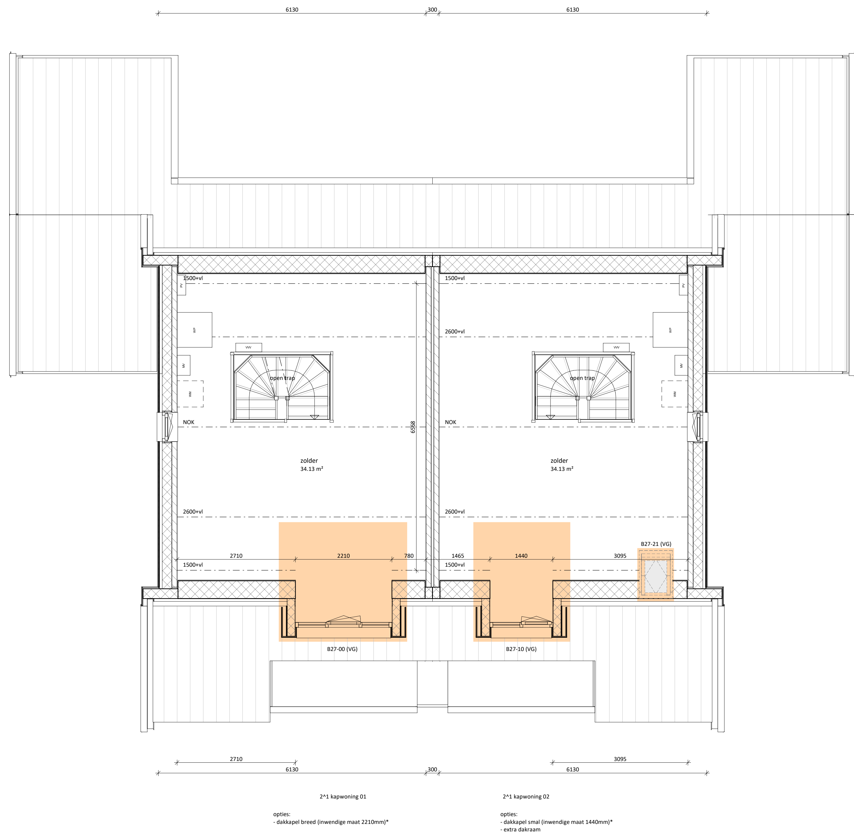
tweede verdieping 1 : 50
