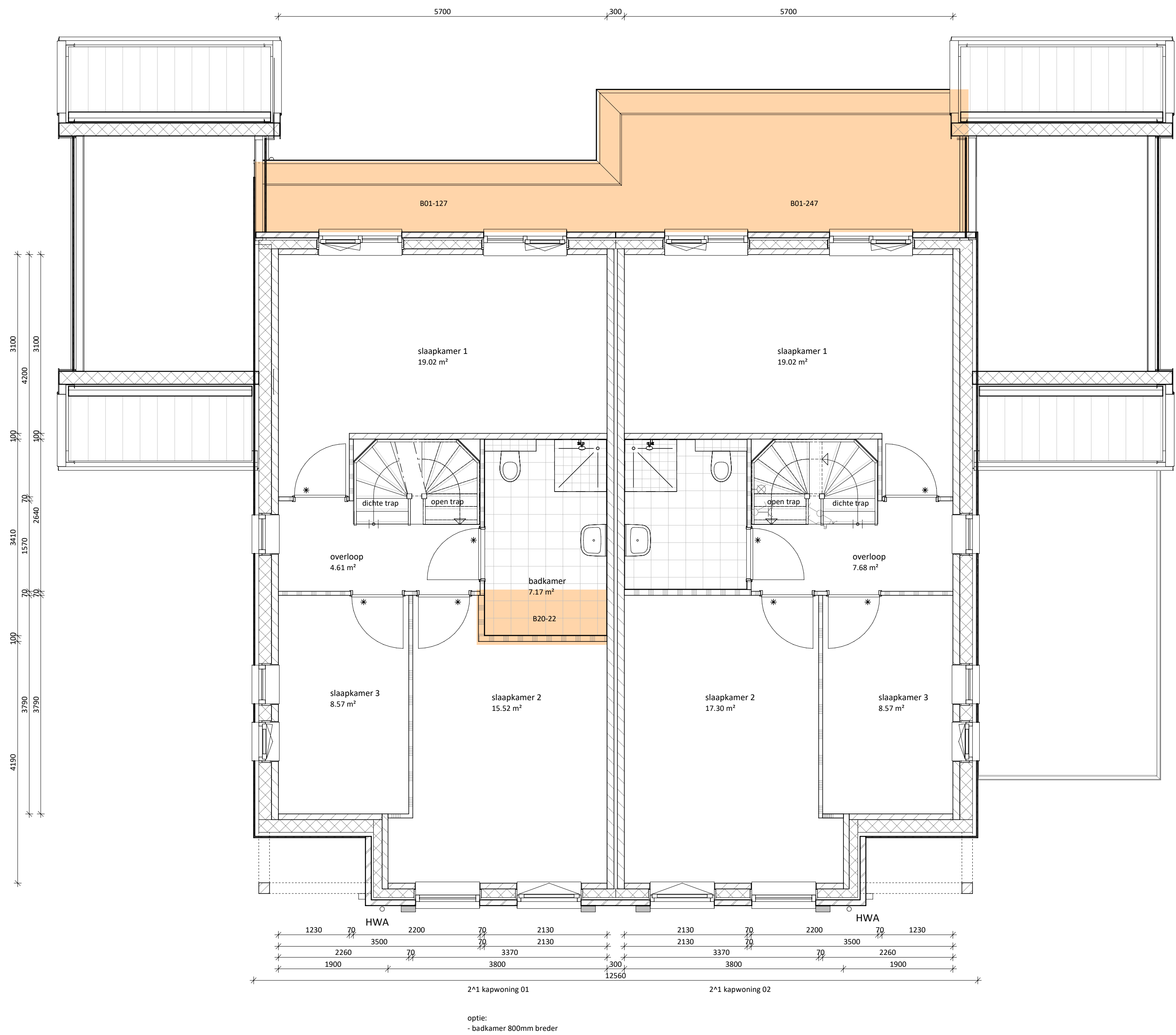
eerste verdieping 1 : 50
