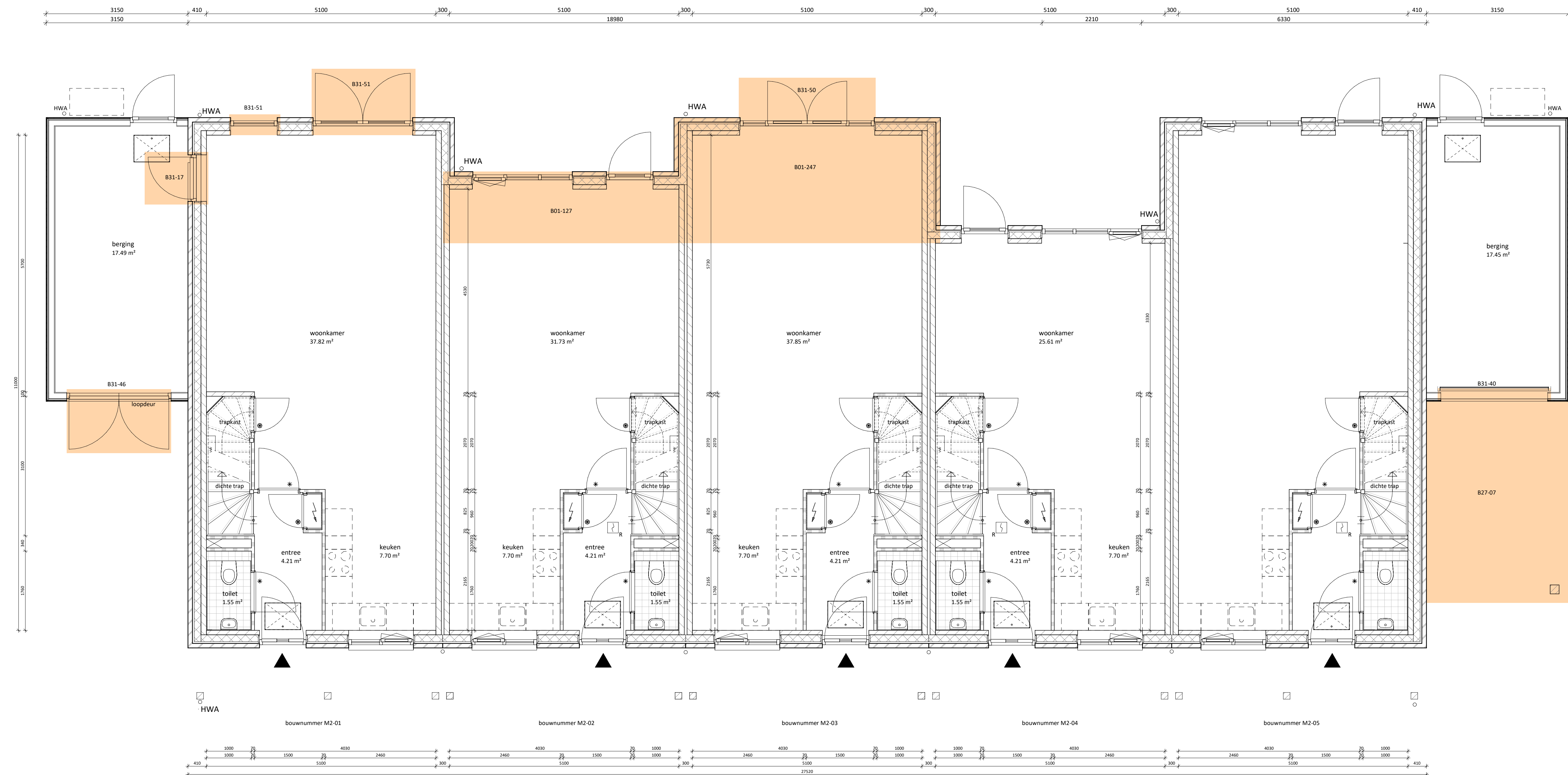
begane grond 1 : 50
