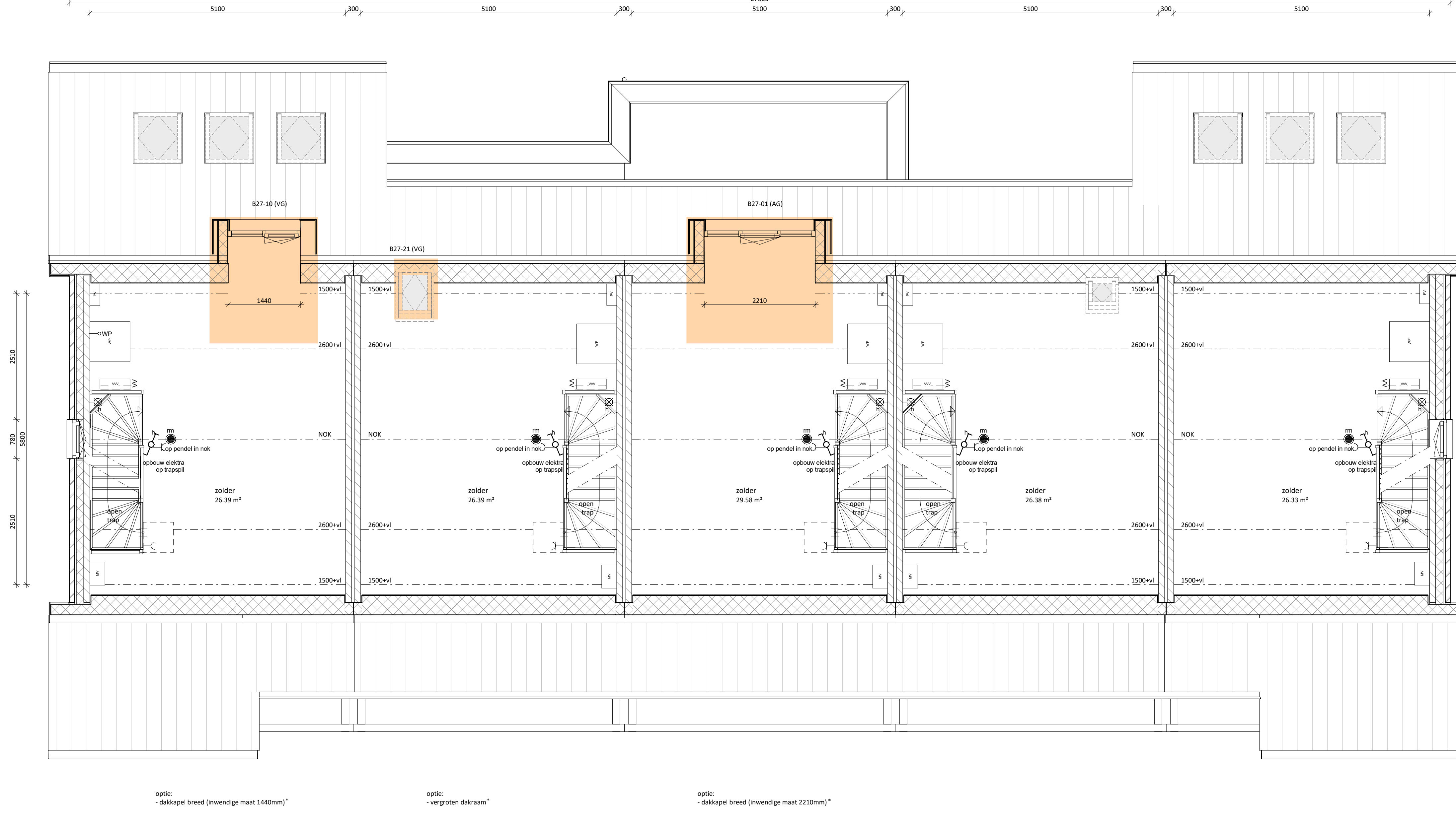
tweede verdieping 1 : 50
