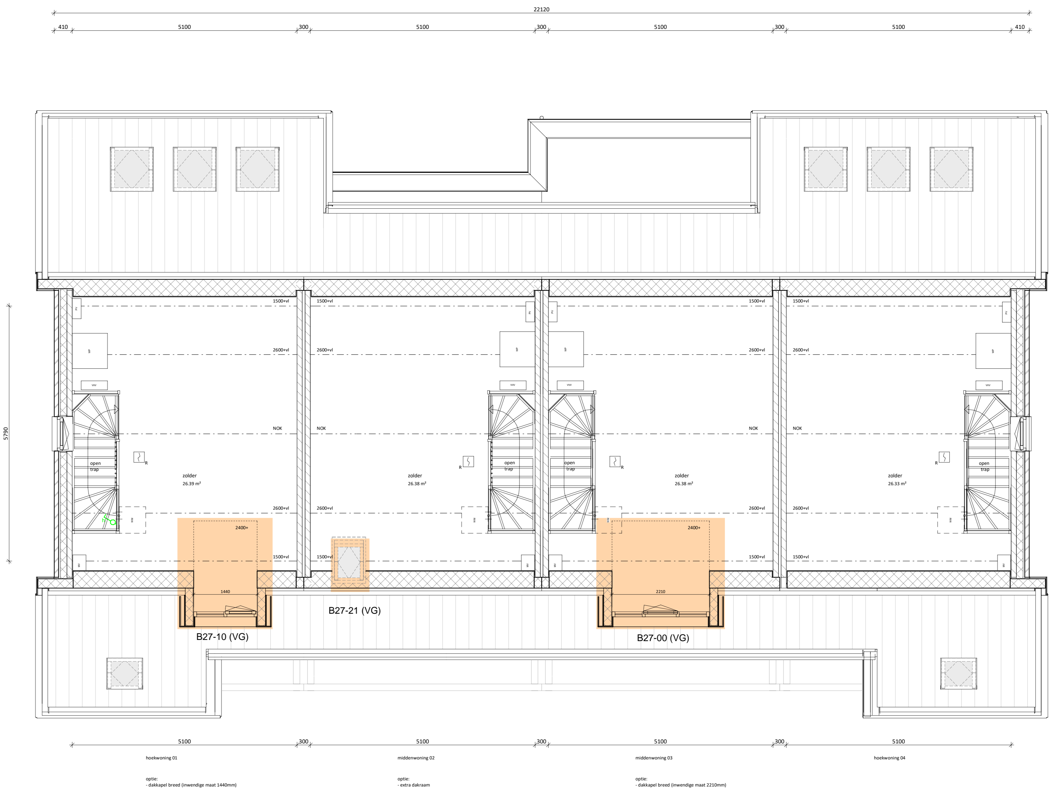
tweede verdieping 1:50
