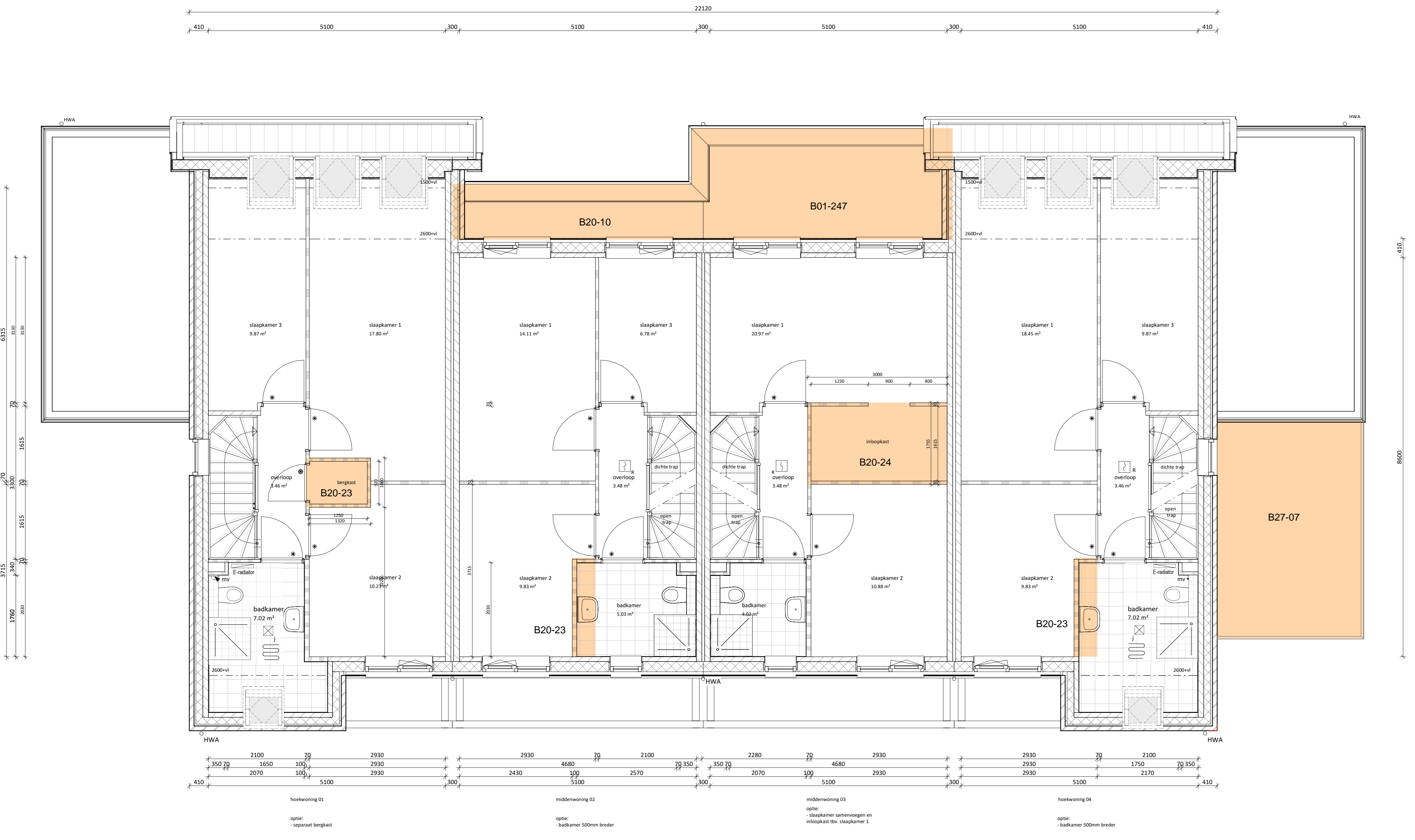
eerste verdieping 1:50
