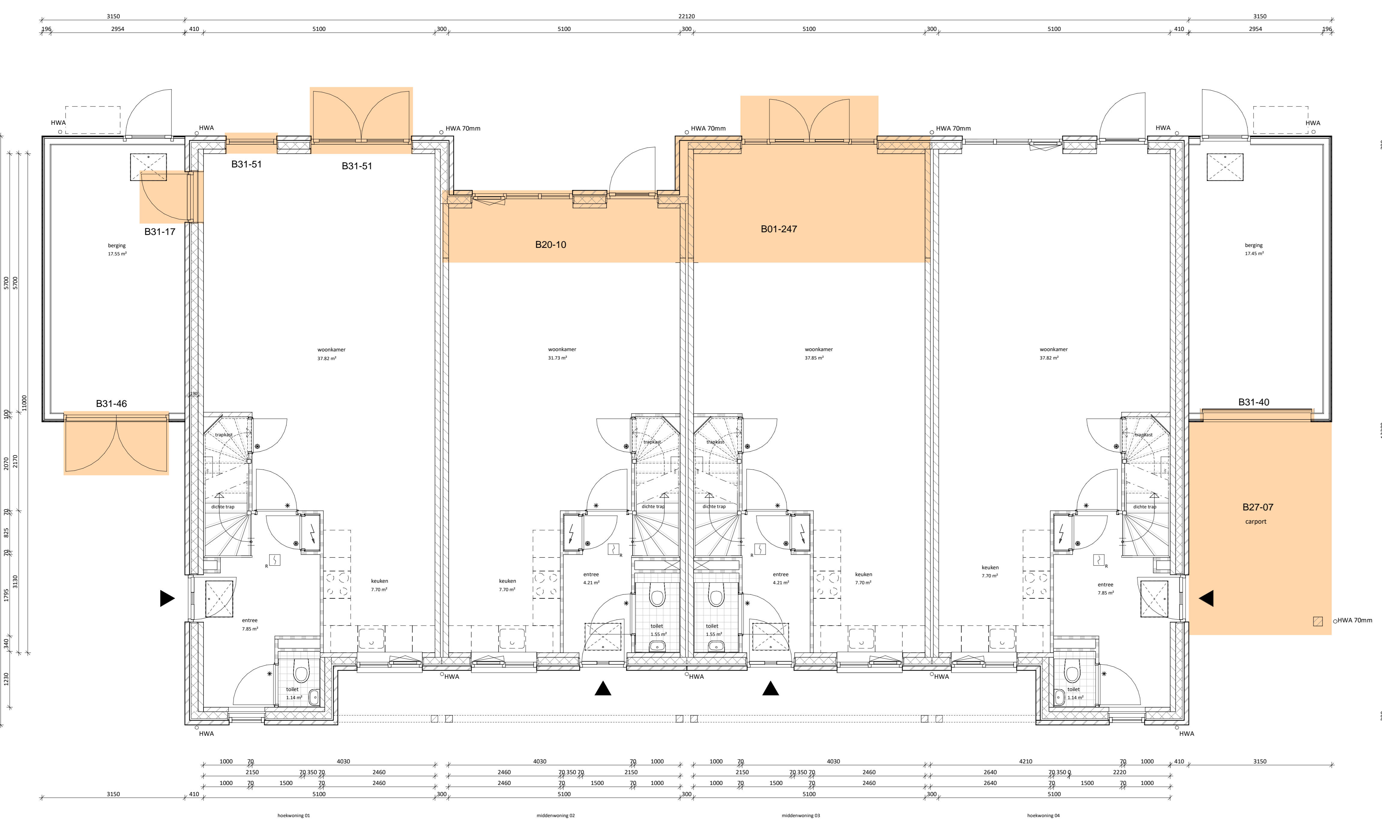
begane grond 1:50
