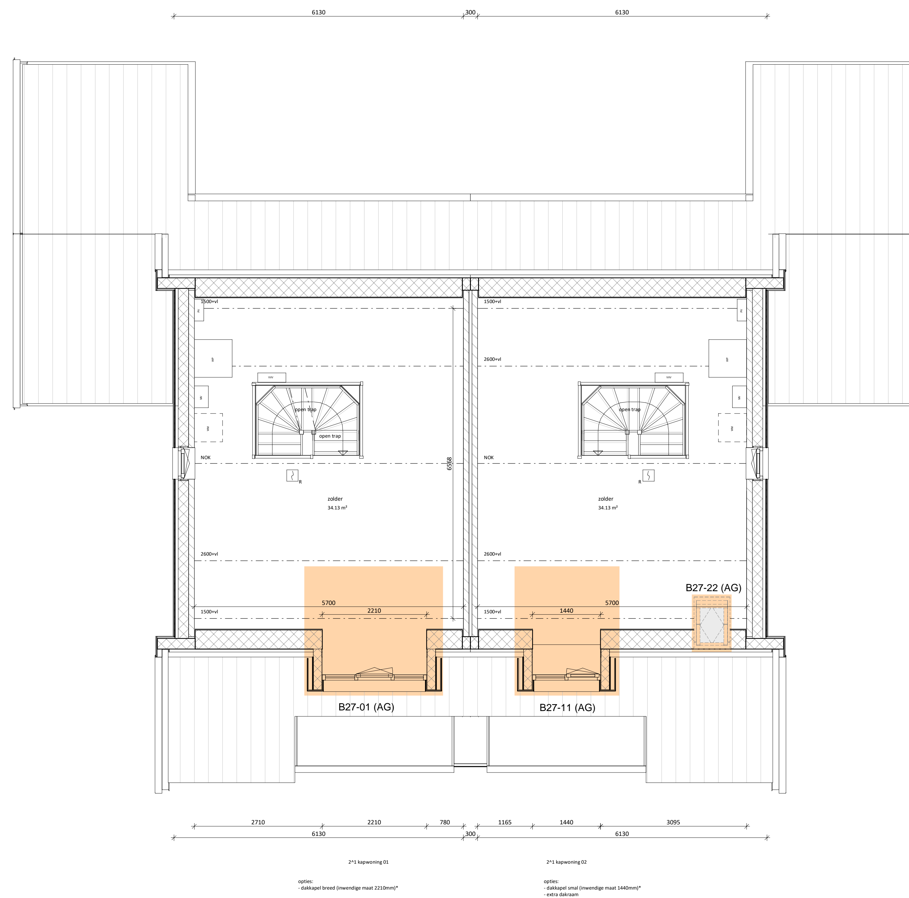
tweede verdieping 1:50
