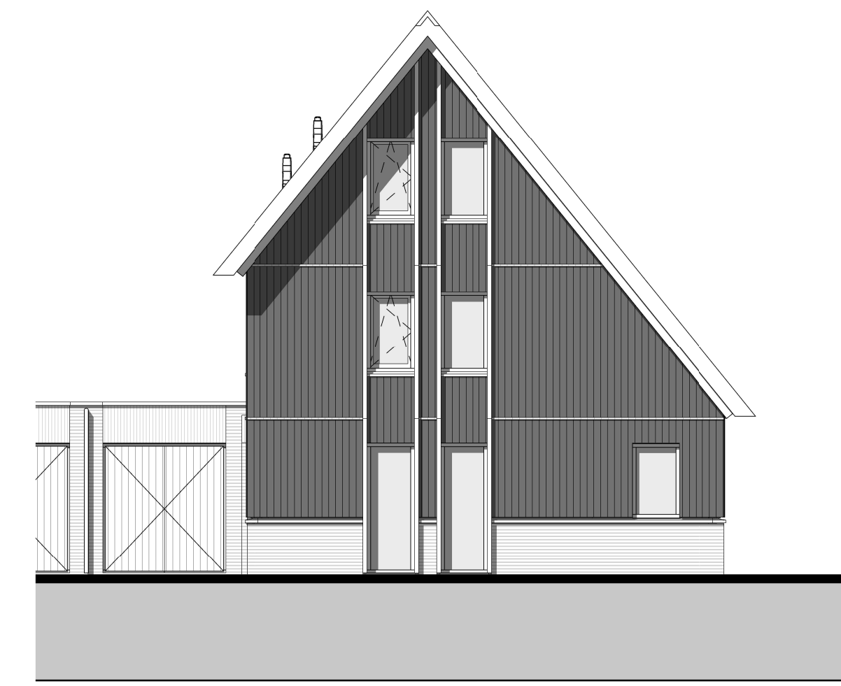
voorgevel 1 : 100
