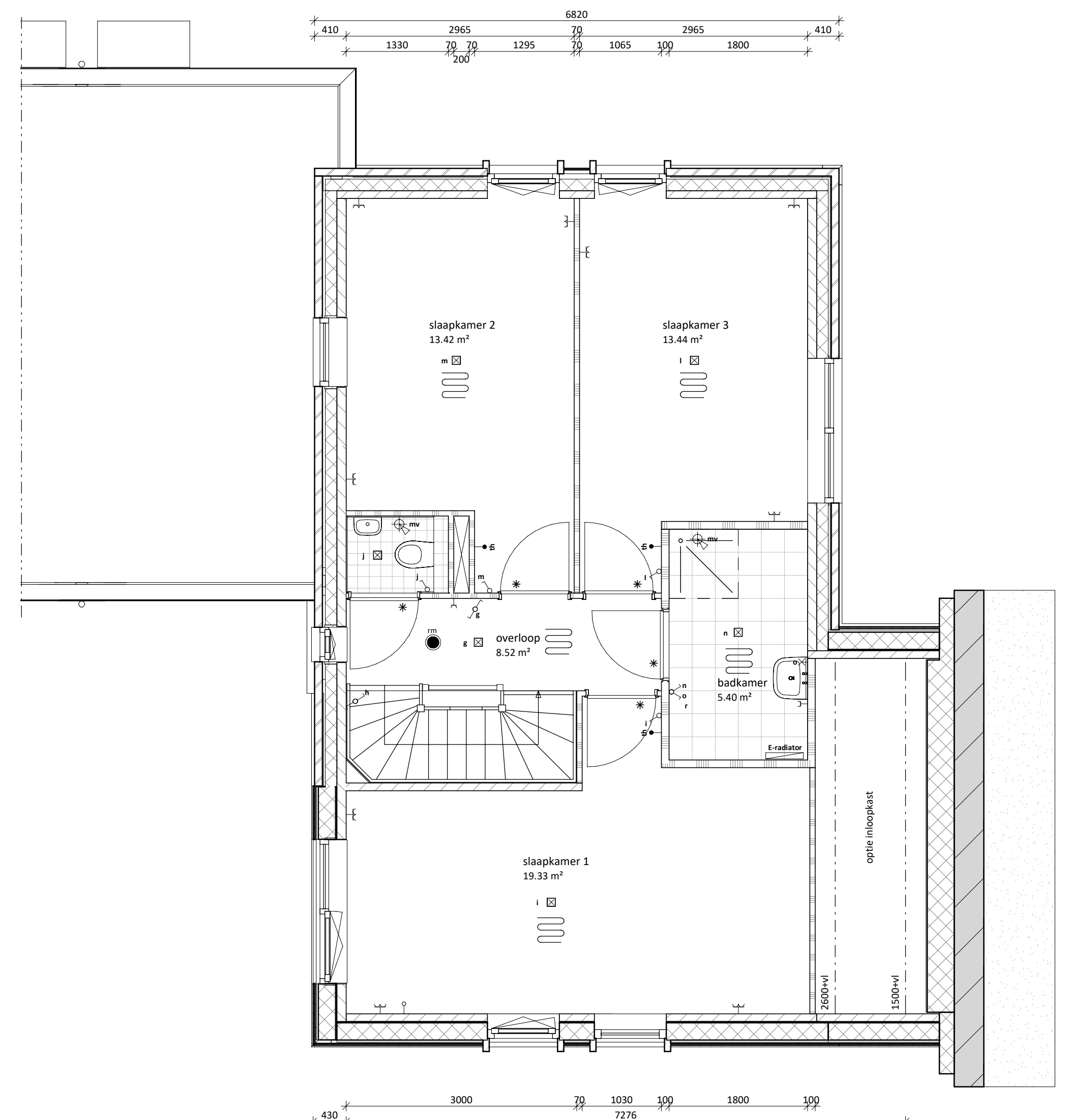
eerste verdieping 1 : 50
