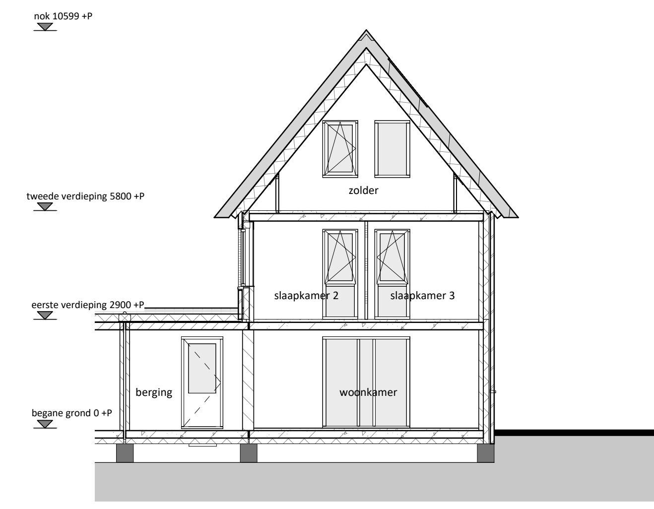
doorsnede 1 : 100
