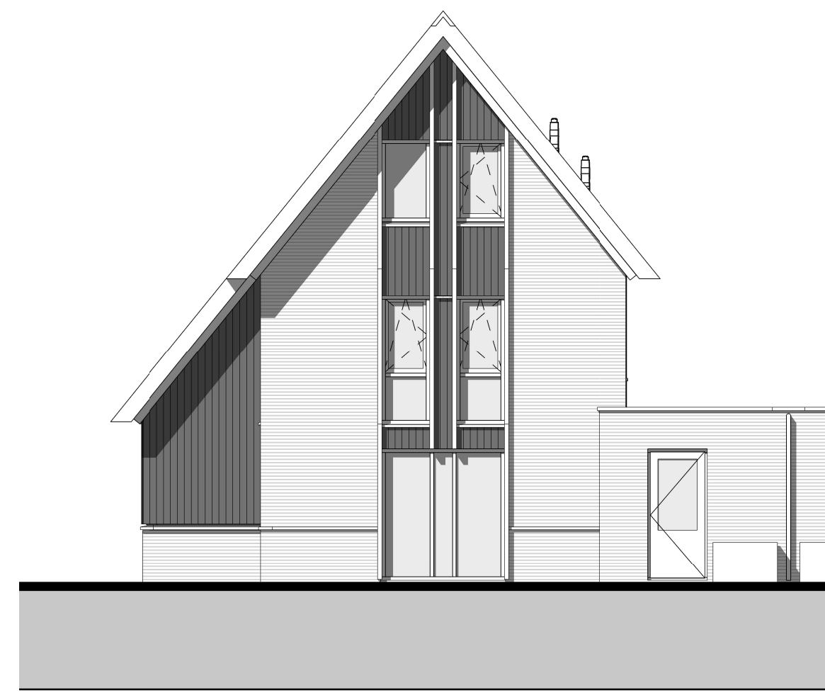
achtergevel 1 : 100
