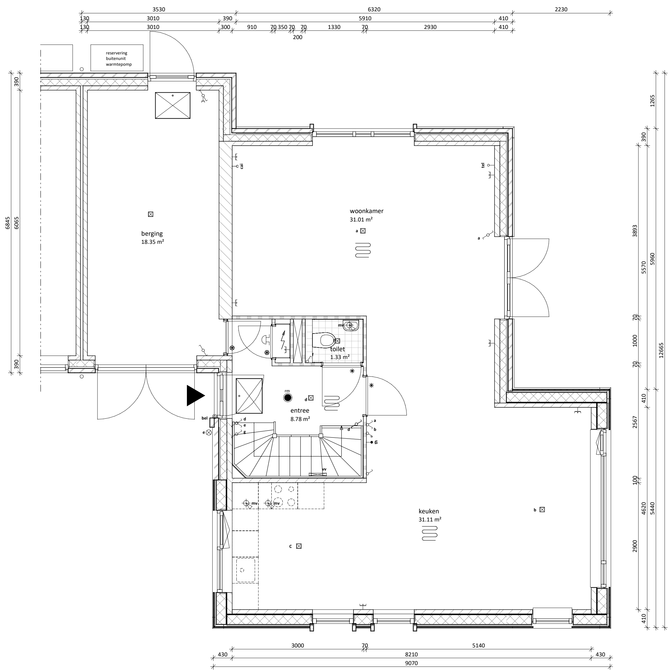
begane grond 1 : 50
