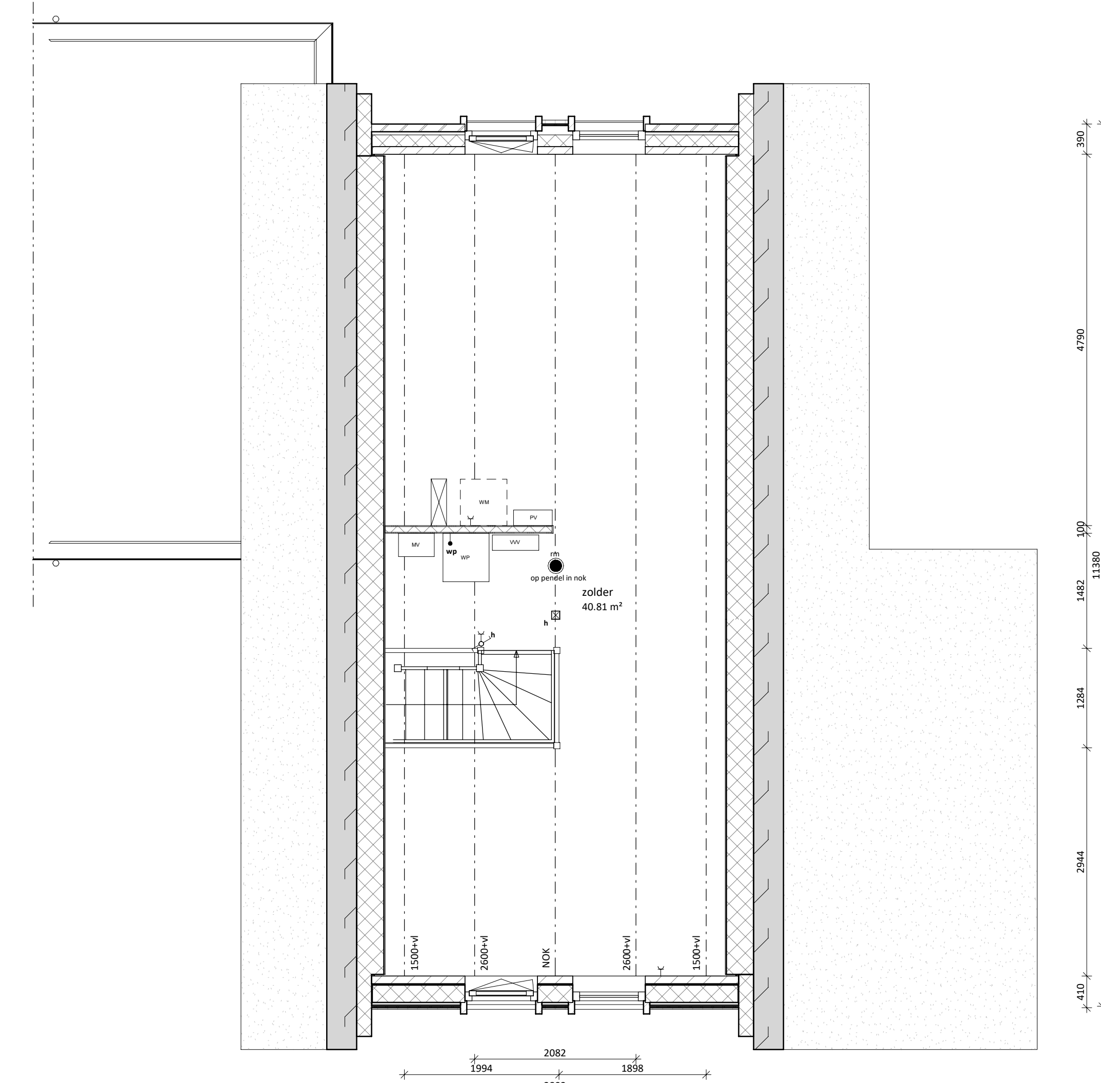
tweede verdieping 1 : 50
