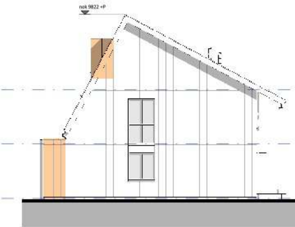
A3 - Linkerzijgevel
